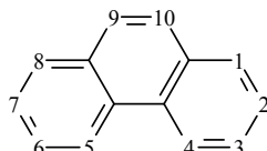
Phénanthrène
