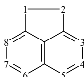
Acenaphthène
