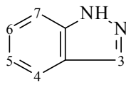
Isoindazole
