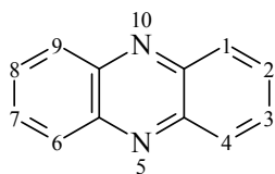
Phénazine
