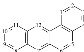
Benzo[a]anthracène
