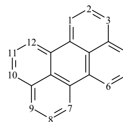
Pérylène
