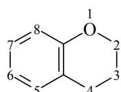
Chromane
