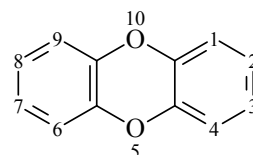
Benzodioxine
