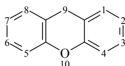
Xanthène
