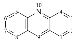
Acridine
