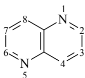
Pyrido[3,2-b]pyridine
