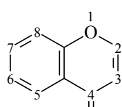
Chromone
