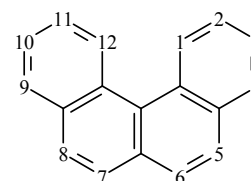
Benzo[c]phénanthrène
