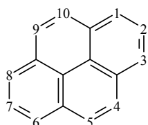
Pyrène
