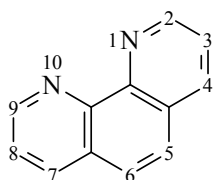
Phénanthroline
