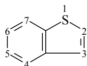
Thionaphtène
