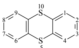
Thianthrène
