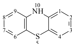
Phénothiazine
