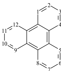
Triphénylène
