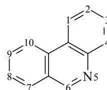
Phénanthridine
