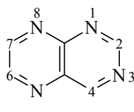
Ptéridine
