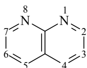
Naphthridine
