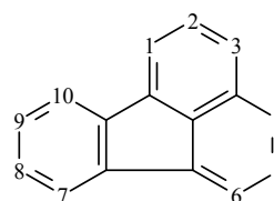
Fluoranthène
