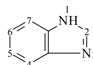
Benzimidazole
