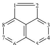
Acenaphthylène
