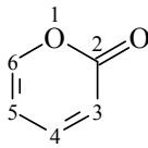
\alpha -Pyrone
