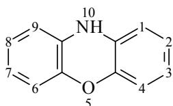
Phénoxazine
