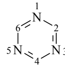
1,2,3-Triazine
